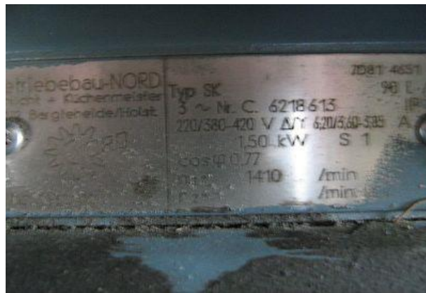
Getriebebau NORD SK 90 L // SK 42125 A-90 L/4
