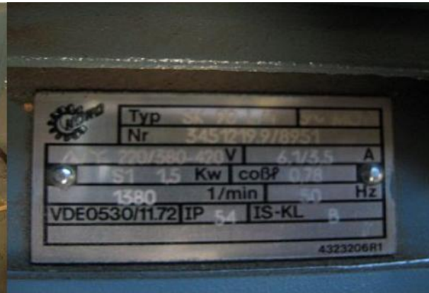
Getriebebau NORD SK 90 L // SK 42125 A-90 L/4
