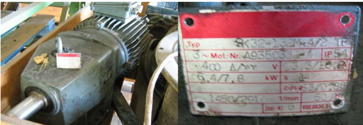
2610 Getriebemotor 6,4/7,8 kW, 400 V/50 Hz, IP 54, Getriebebau NORD SK 32-132 M/4-2 TF
